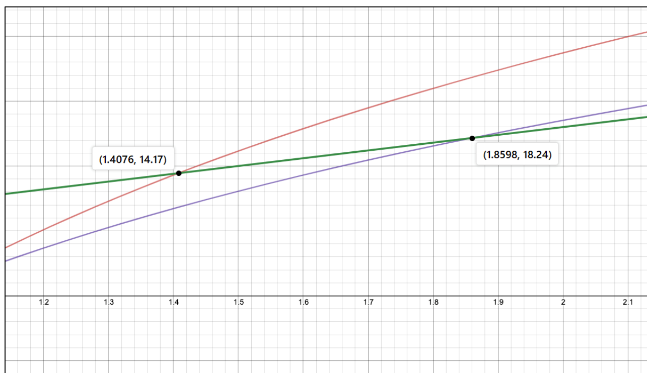
Рисунок 3. Решения систем уравнений.
